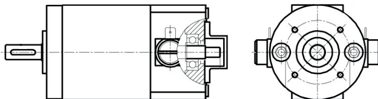
Eksempel på snittegning af PENTA DC-motor 1S/1M/1L.
